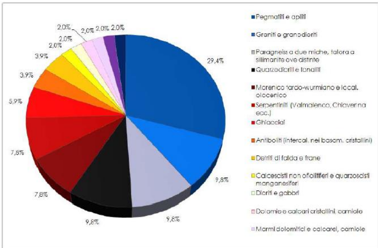
Рисунок 31. Состав геологического субстрата в зоне ZPS (%). (25)
