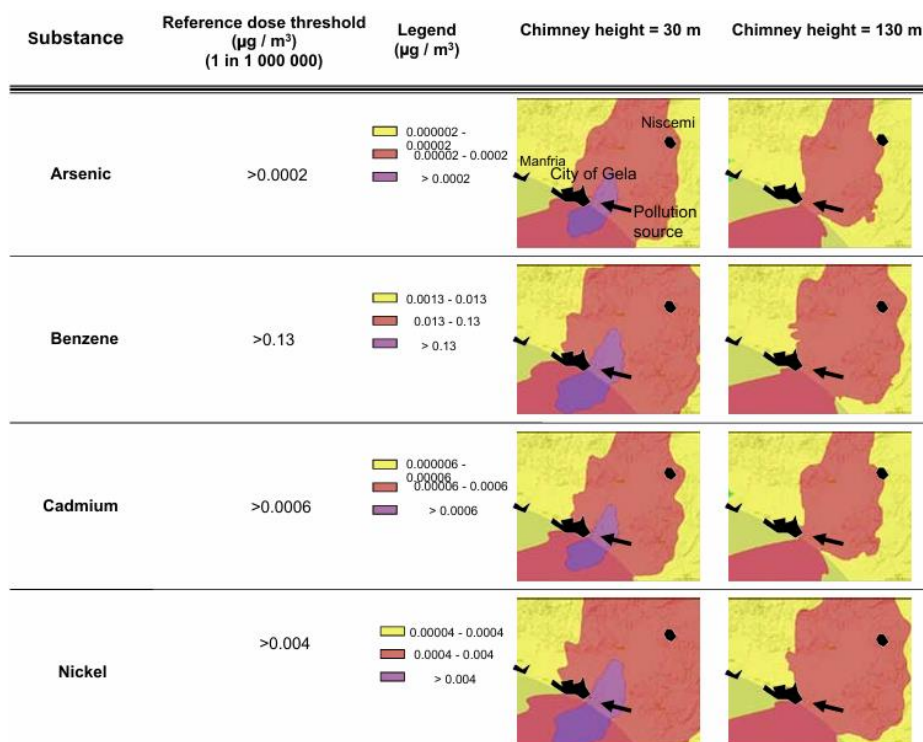
Рисунок 15. Концентрации мышьяка, бензола, кадмия и никеля , рассчитанные с использованием модели дисперсии METI-LIS.
